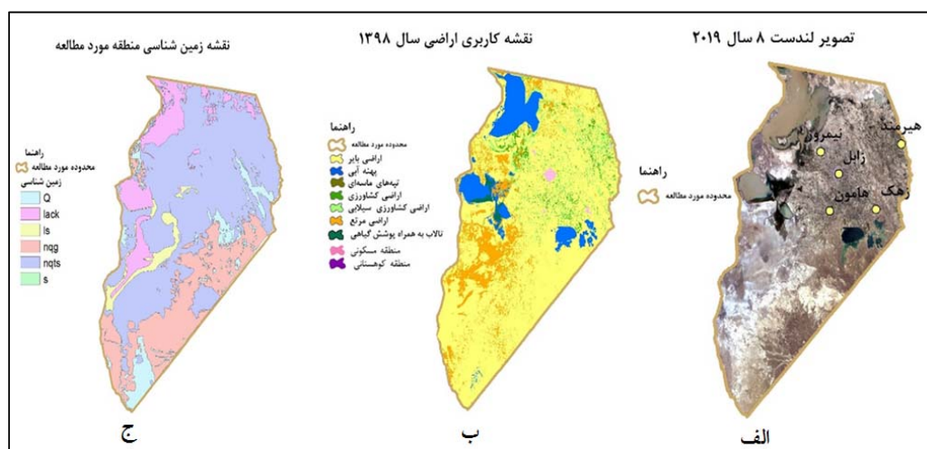
شکل ۳- تصاویر سنجنده OLI ماهواره لندست هشت (الف)، نقشه کاربری اراضی (ب)، نقشه زمین‌شناسی (ج)
