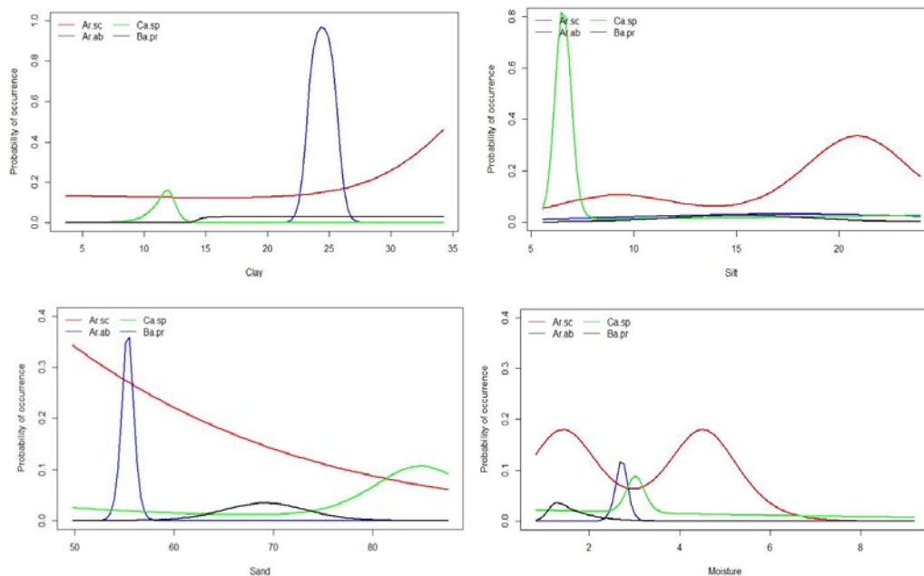
شکل ۱- مدل‌سازی پاسخ چهار گیاه بوته‌ای به بافت و رطوبت باطله زغال‌سنگ در معدن کارمزد سوادکوه، استان مازندران
