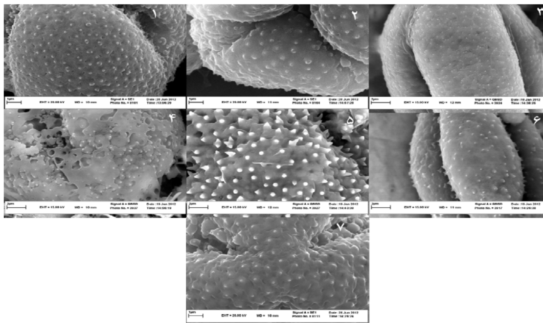
شکل ۳- تصویر میکروسکوپ الکترونی ریزساختار سطح دانه گرده گونه‌های مورد مطالعه جنس Cuscuta در شمال شرق ایران. ۱: C. pedicellata ، ۲: C. kotschyana ، ۳: C. brevistyla ، ۴: C. campestris ، ۵: C. monogyna ، ۶: C. babylonica var. babylonica ، ۷: C. pedicellata بزرگنمایی 25000x.
