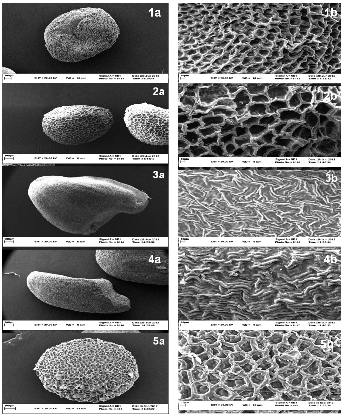
شکل ۴- تصاویر بذر پنج گونه از جنس Cuscuta در مطالعه با میکروسکوپ الکترونی نگاره: ۱: C. campestris ، ۲: C. epithymum ، ۳: C. monogyna ، ۴: C. lehmanniana var. lehmanniana ، ۵: C. babylonica var. babylonica
