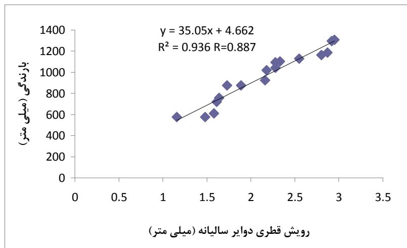
شکل ۴- رابطه میانگین رویش قطری دایره سالیانه با بارندگی در رویشگاه ۳
