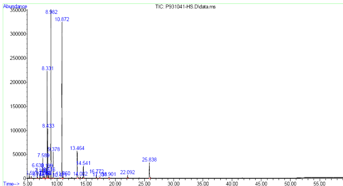
شکل ۱- کروماتوگرام اسانس گل نرگس به روش میکرو استخراج فاز جامد در فضای فوقانی
