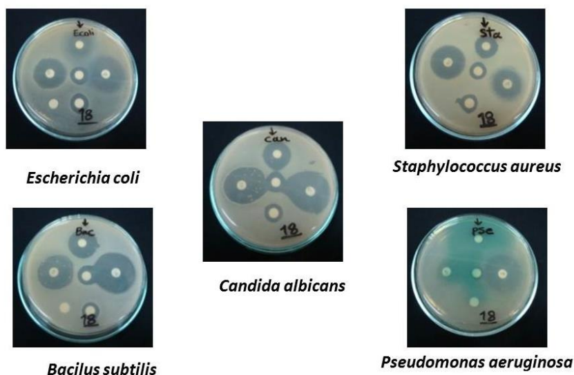
شکل ۲ - هاله های ممانعت از رشد ایجاد شده توسط اسانس Thymus Fedchenkoii از استان سمنان با روش انتشار از دیسک
