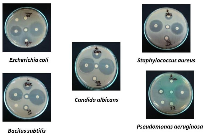
شکل ۱ - هاله‌های ممانعت از رشد ایجاد شده توسط اسانس Thymus fedtschenkoi از استان زنجان با روش انتشار از دیسک
