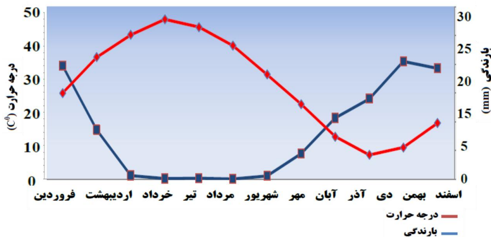
شکل ۱- نمودار آمبروترمیک ایستگاه هواشناسی سینوپتیک فرودگاه بیرجند
