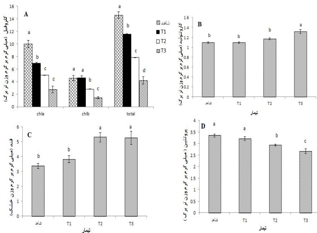
شکل ۲- میانگین کلروفیل (A)، کاروتنوئید (B)، قند (C) و پروتئین (D) در شدت‌های متفاوت تابش فرابنفش. (۰:شاهد، T1: ۰/۱۲، T2: ۰/۲۶ و T3: ۰/۳۸ وات بر مترمربع). نتایج میانگین سه تکرار ( Maen \pm SE ) را نشان می‌دهد. حروف متفاوت نشان دهنده معنی دار بودن تفاوت‌ها در سطح ( P \leq 0.05 ) براساس آزمون دانکن می‌باشند.
