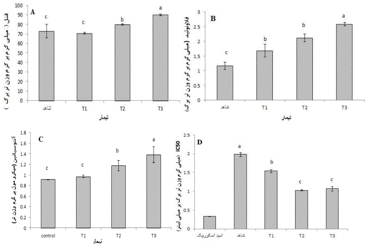
شکل ۱- میانگین فنل کل (A)، فلاونوئید (B)، آنتوسیانین (C) و IC_{50} (D) عصاره متانولی در شدت‌های متفاوت تابش فرابنفش. (شاهد، T1: 0/12 وات بر مترمربع). نتایج میانگین سه تکرار ( Maen \pm SE ) را نشان می‌دهد. حروف متفاوت نشان‌دهنده معنی‌دار بودن تفاوت‌ها در سطح ( P \leq 0/05 ) براساس آزمون دانکن می‌باشند.
