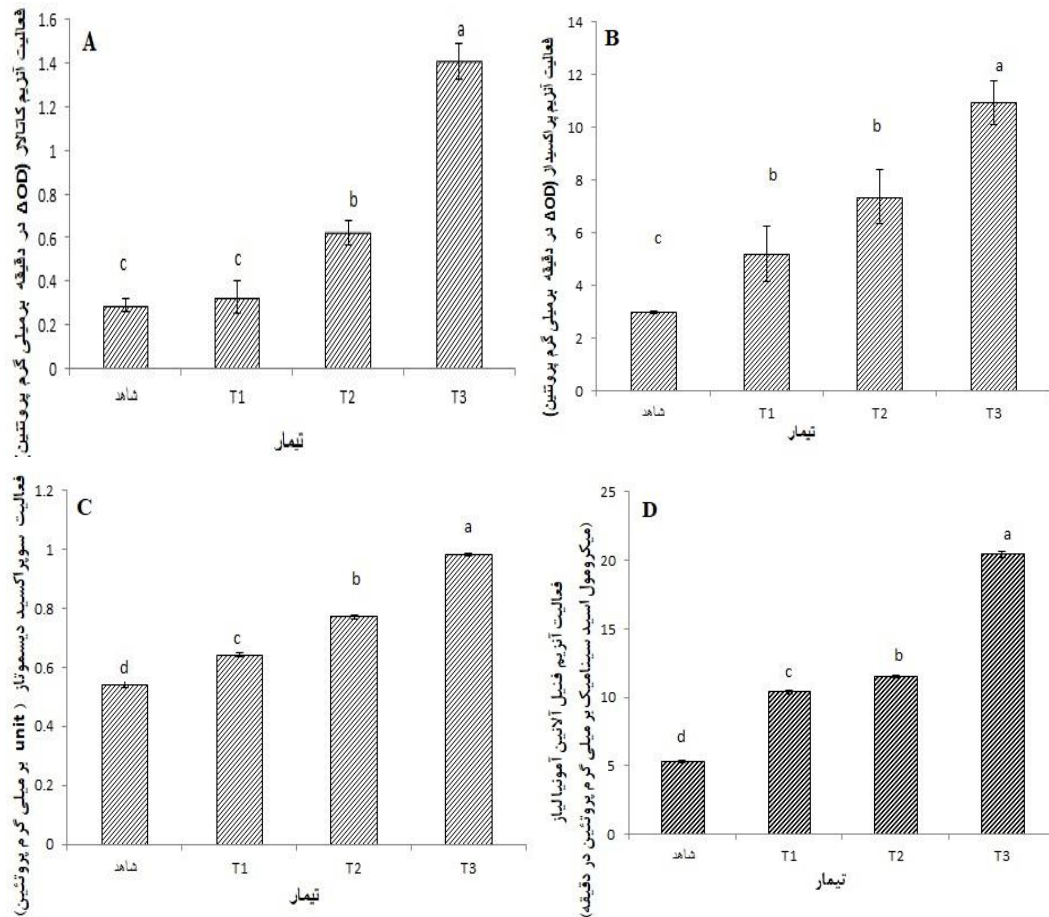
شکل ۳- فعالیت آنزیم‌های کاتالاز (A)، پراکسیداز (B)، سوپراکسید دیسموتاز (C) و فنیل آلانین آمونیا لیااز (D) در شدت‌های متفاوت تابش فرابنفش. (شاهد: ۰، T1: ۰/۱۲، T2: ۰/۲۶، T3: ۰/۳۸ وات بر مترمربع). نتایج میانگین سه تکرار (Mean±SE) را نشان می‌دهد. حروف متفاوت نشان‌دهنده معنی‌دار بودن تفاوت‌ها در سطح ( P \leq 0/05 ) بر اساس آزمون دانکن می‌باشند.
