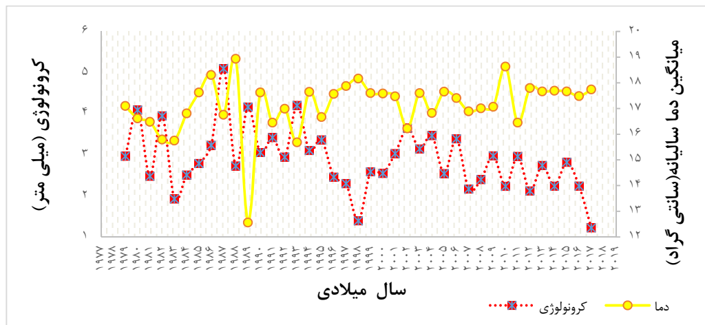
شکل ۷- نمودار کرونولوژی- دما درختان زربین منطقه رودبار، در دوره رویشی ۱۹۷۹ تا ۲۰۱۷
