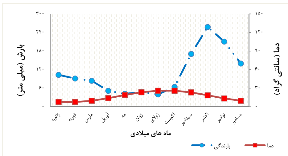
شکل ۳- منحنی آمبروترمیک ایستگاه هواشناسی نوشهر (۱۹۷۷-۲۰۱۷)
