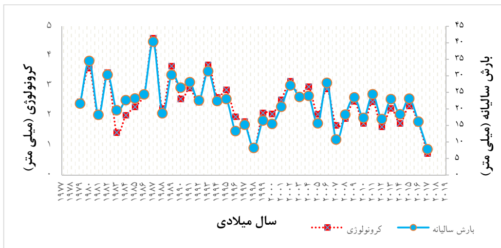
شکل ۶- نمودار کرونولوژی- بارش درختان زربین منطقه رودبار در دوره رویشی ۱۹۷۹ تا ۲۰۱۷
