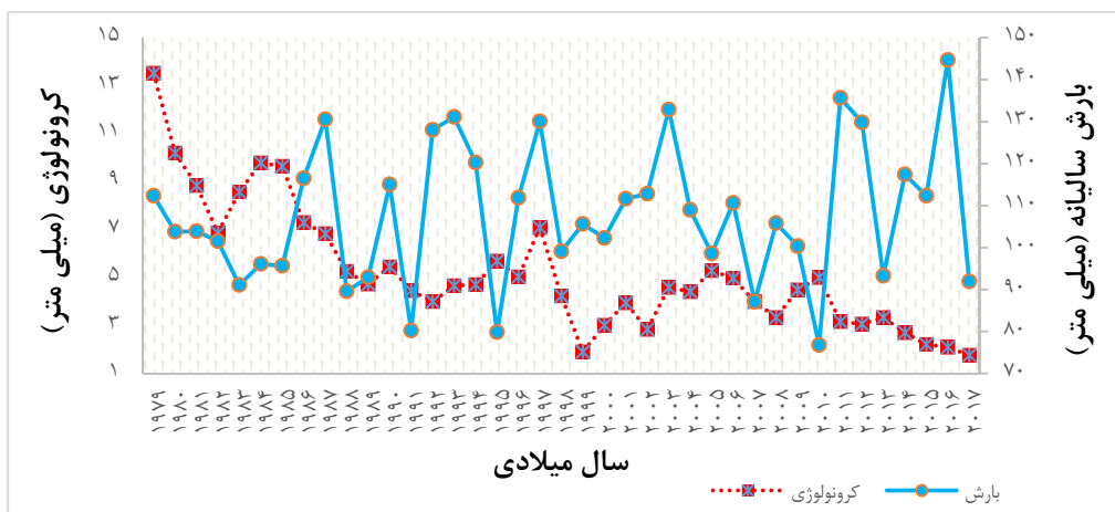
شکل ۸- نمودار کرونولوژی- بارش درختان زربین در منطقه نوشهر در دوره رویشی ۱۹۷۹ تا ۲۰۱۷
