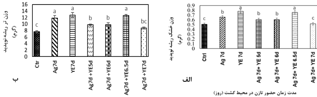
شکل ۳- تأثیر تیمارهای انفرادی و ترکیبی نیترات نقره و عصاره مخمر بر وزن تر (الف) و وزن خشک (ب) ریشه‌های نوپدید P. abrotanoides . داده‌ها میانگین سه تکرار \pm انحراف معیار هستند. براساس آزمون دانکن، حروف یکسان نشان دهنده عدم تفاوت معنی‌دار ( P > 0.05 ) می‌باشند. Ag: نیترات نقره با غلظت 25 \mu\text{M} ; YE: عصاره مخمر با غلظت 200 \text{ mg/L} ; d: مدت زمان حضور تازن در محیط کشت (روز)
