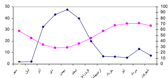
شکل ۱- منحنی آمبروترمیک ایستگاه سرچاهان (۹۵-۱۳۷۵)
