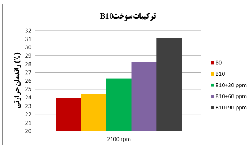
شکل ۴- راندمان حرارتی موتور دیزل در دور ۲۱۰۰ rpm.
