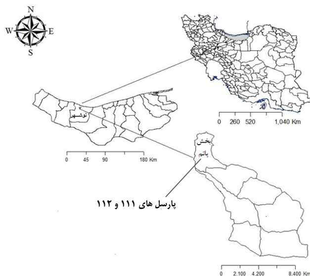
شکل ۲- منطقه مورد مطالعه بخش پاتم جنگل خیرود
