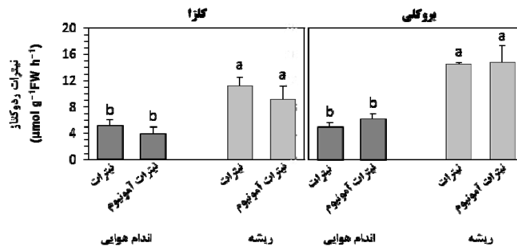
نمودار ۴ - تاثیر نیترات و نیترات آمونیوم بر فعالیت آنزیم نیترات ردوکتاز در ریشه و اندام هوایی گیاهچه های کلزا و بروکلی. میانگین های دارای حروف لاتین غیر مشابه بر اساس آزمون واریانس یک سویه در سطح احتمال یک درصد معنی دار هستند ( p < 0.01 ).
