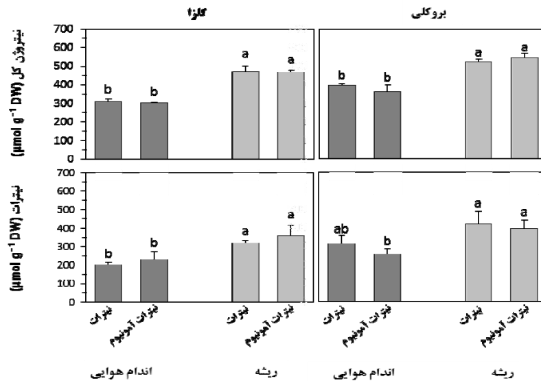
نمودار ۳ - تاثیر نیترات و نیترات آمونیوم بر محتوای نیتروژن کل و نیترات در ریشه و اندام هوایی گیاهچه های کلزا و بروکلی. میانگین های دارای حروف لاتین غیر مشابه بر اساس آزمون واریانس یک سویه در سطح احتمال یک درصد معنی دار هستند ( p < 0.01 ).
