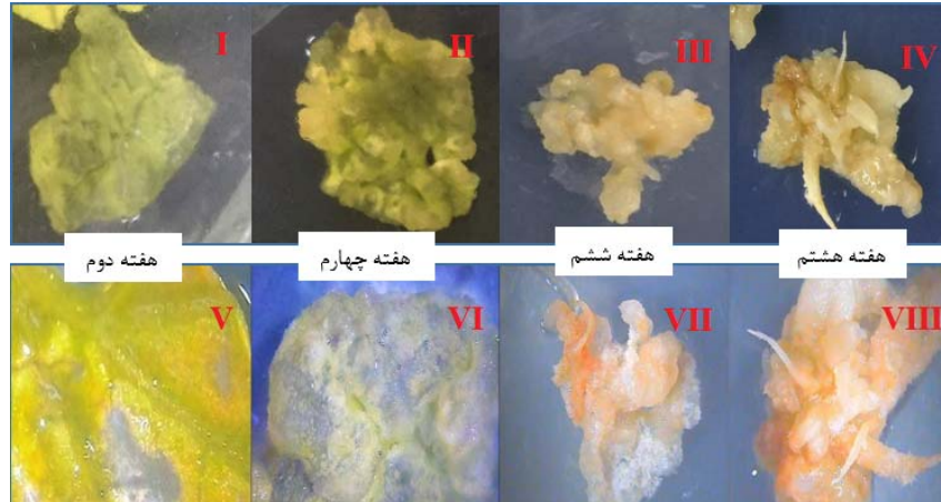
شکل ۳- مراحل مختلف تشکیل کالوس و ریشه بر روی برگ در حالی که سطح بالایی ریزنمونه برگ خربزه تلخ در تماس با محیط کشت MS حاوی NAA بوده است. تصاویر I, II, III, IV، نمای ماکروسکوپی مربوط به استقرار سطح بالایی برگ بروی محیط کشت حاوی ۲ mg/l NAA تحت شرایط تاریکی که به ترتیب از هفته دوم، چهارم، ششم و هشتم تهیه شده است. (نمای ماکروسکوپی با دوربین دیجیتال کانن مدل Powershot SX60 HS تهیه شده است) و تصاویر V, VI, VII, VIII نمای میکروسکوپی مربوط به استقرار سطح بالایی برگ بروی محیط کشت حاوی ۲ mg/l NAA تحت شرایط تاریکی که به ترتیب از هفته دوم، چهارم، ششم و هشتم تهیه شده است. (نمای میکروسکوپی با دوربین Color Video Camera Sony مدل SSD-DC58AP که روی بیناکولار Olympus قرار گرفته و در بزرگنمایی 100x تهیه شده است).
