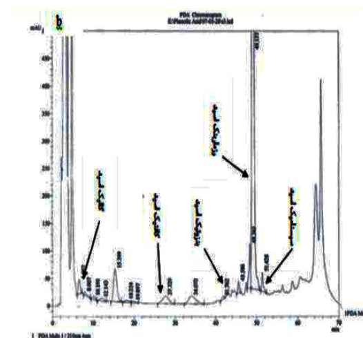
شکل ۸- منحنی کروماتوگرام حاصل از HPLC مقدار اسیدهای فنلی (a منحنی استاندارد و b منحنی نمونه)
