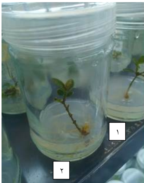
شکل ۵- اثر غلظت‌های مختلف BAP و IBA روی طول ریشه در گیاهچه‌های شمشاد خزری ( Buxus hyrcana Pojark.) رشدیافته در شرایط درون‌شیشه‌ای. (۱) گیاهچه‌های شاهد و (۲) گیاهچه‌های تیمارشده با ۰/۵ میلی‌گرم در لیتر BAP همراه با ۱/۵ میلی‌گرم در لیتر IBA.
