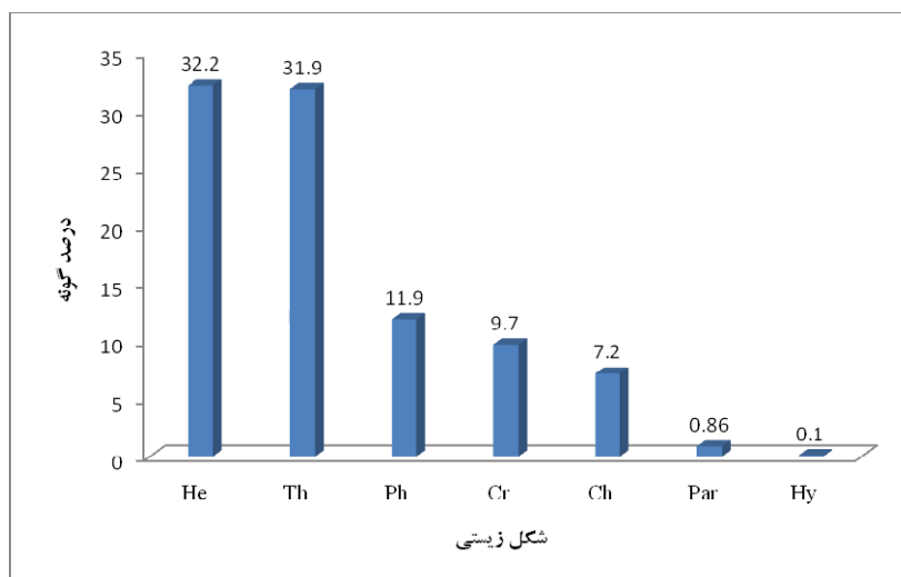
نمودار ۴- درصد فراوانی شکل‌های زیستی گیاهان منطقه حفاظت شده قمصر (Ch: کامفیت‌ها، Cr: کریپتوفیت‌ها (ژئوفیت‌ها)، He: همی کریپتوفیت‌ها، Ph: فانروفیت‌ها، Th: تروفیت‌ها).
