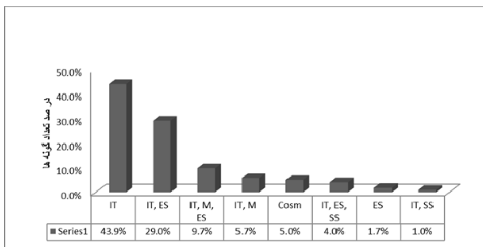
شکل ۴- سهم عناصر نواحی رویشی مختلف ایران در پوشش گیاهی منطقه مورد مطالعه. ایرانی‌تورانی (IT، مدیترانه‌ای (M)، اروپایی سبیریایی (ES)، صحاری‌سندی (SS) و جهان وطنی (Cosm).
