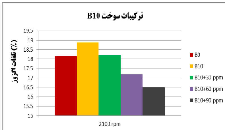
شکل ۶- تلفات حرارتی اگزوز موتور دیزل در دور ۲۱۰۰ rpm.
