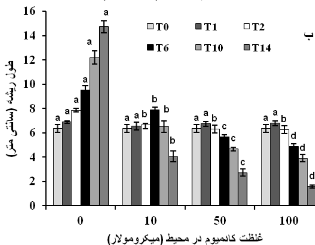
شکل ۳- تاثیر غلظت‌های مختلف کادمیوم (۰، ۱۰، ۵۰ و ۱۰۰ بر حسب میکرومولار) بر طول اندام هوایی و (ب) ریشه. مقادیر میانگین سه تکرار \pm SD می‌باشند. در هر برداشت زمانی حروف غیر مشترک بیانگر وجود تفاوت معنی‌دار بین غلظت‌های مختلف کادمیوم در سطح احتمال ۵ درصد می‌باشند.
